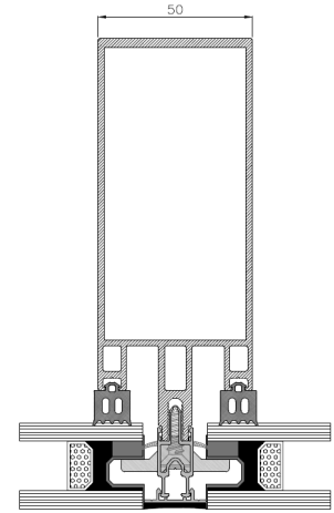
Sección montante
