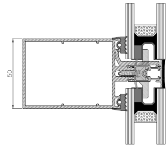
Sección travesaño
