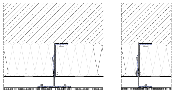
Sección horizontal.
