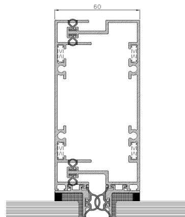
Sección montante
