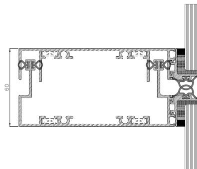
Sección travesaño
